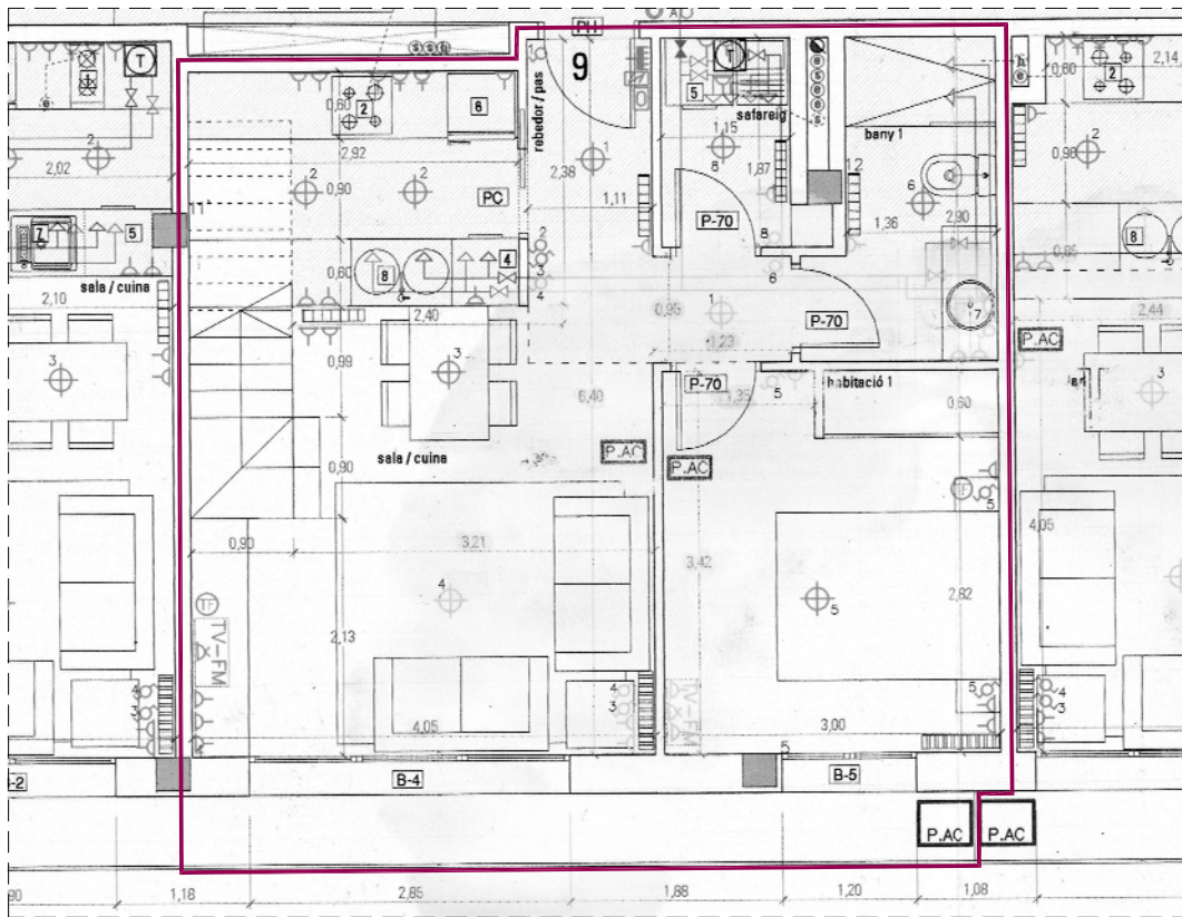
PLANTA SEGONA
